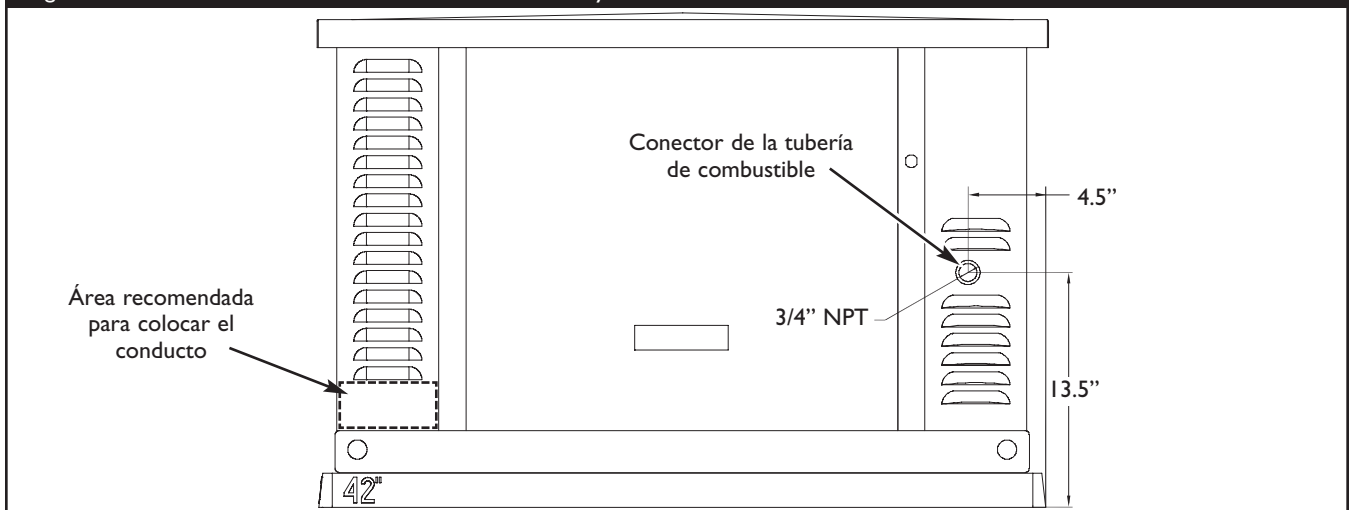
Figura 16 — Ubicaciones de los Accesorios del Conducto y Combustible del Generador, del Lado del Servicio de Aceite de la Unidad
